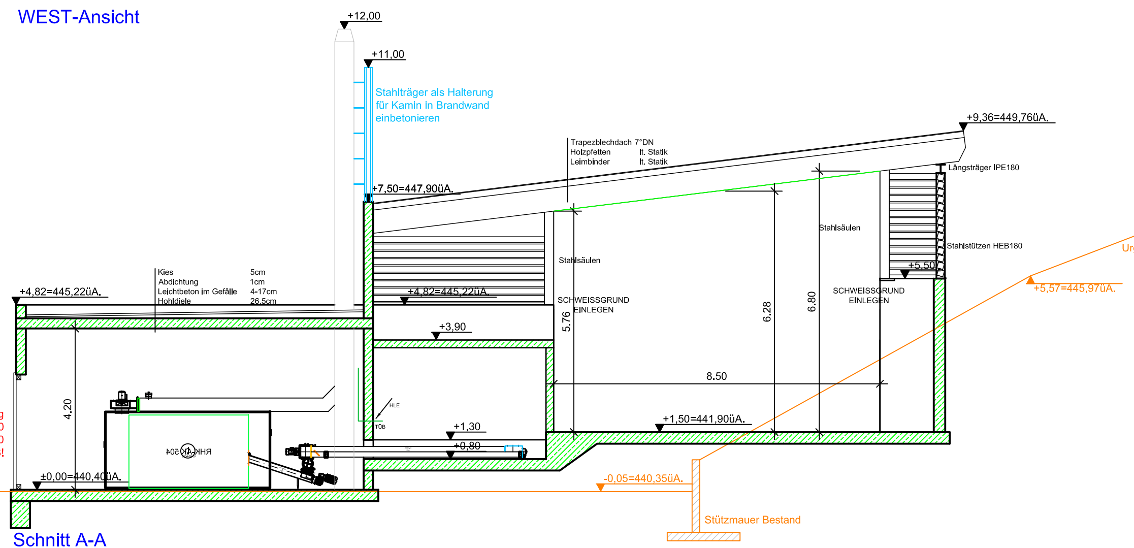
Schnitt A-A
