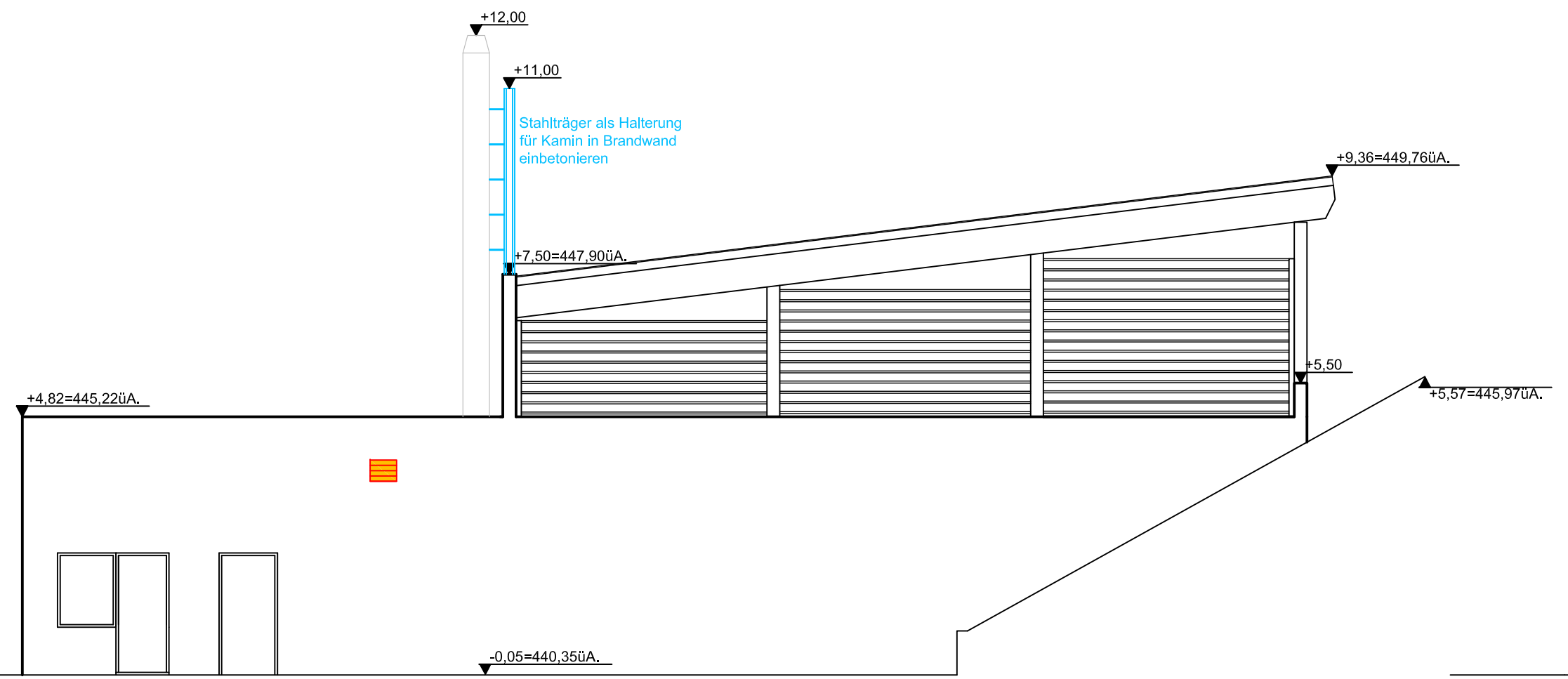
WEST-Ansicht
